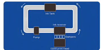
화이트 잉크 순환 시스템으로 헤드 막힘 방지
